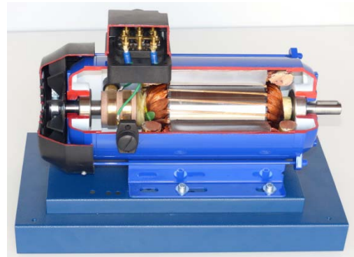
MOD.3070 Machine synchrone triphasée Moteur/alternateur
